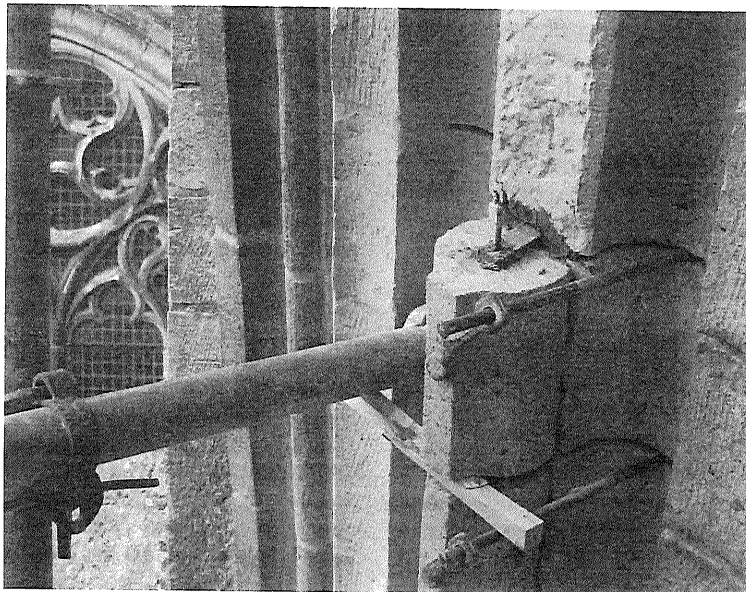
* Gedeeltelijke vervanging van tufstenen neggeblokken in een raam van de Domkerk, bij de zuidgevel van het hoogkoor (foto Van Hoogevest Architecten).
